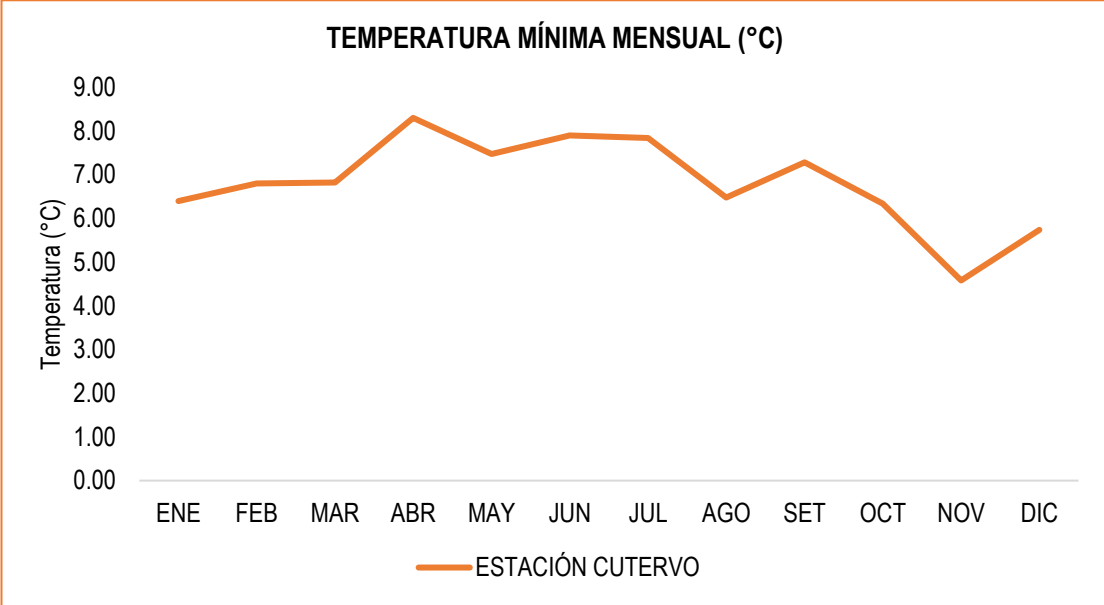
Gráfico 6: Régimen de Temperatura Mínima Media Mensual (°C)
