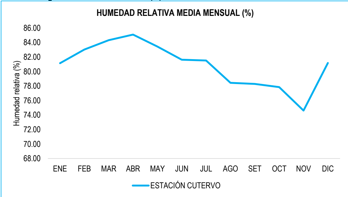
Gráfico 8: Régimen de Humedad Relativa (%)
