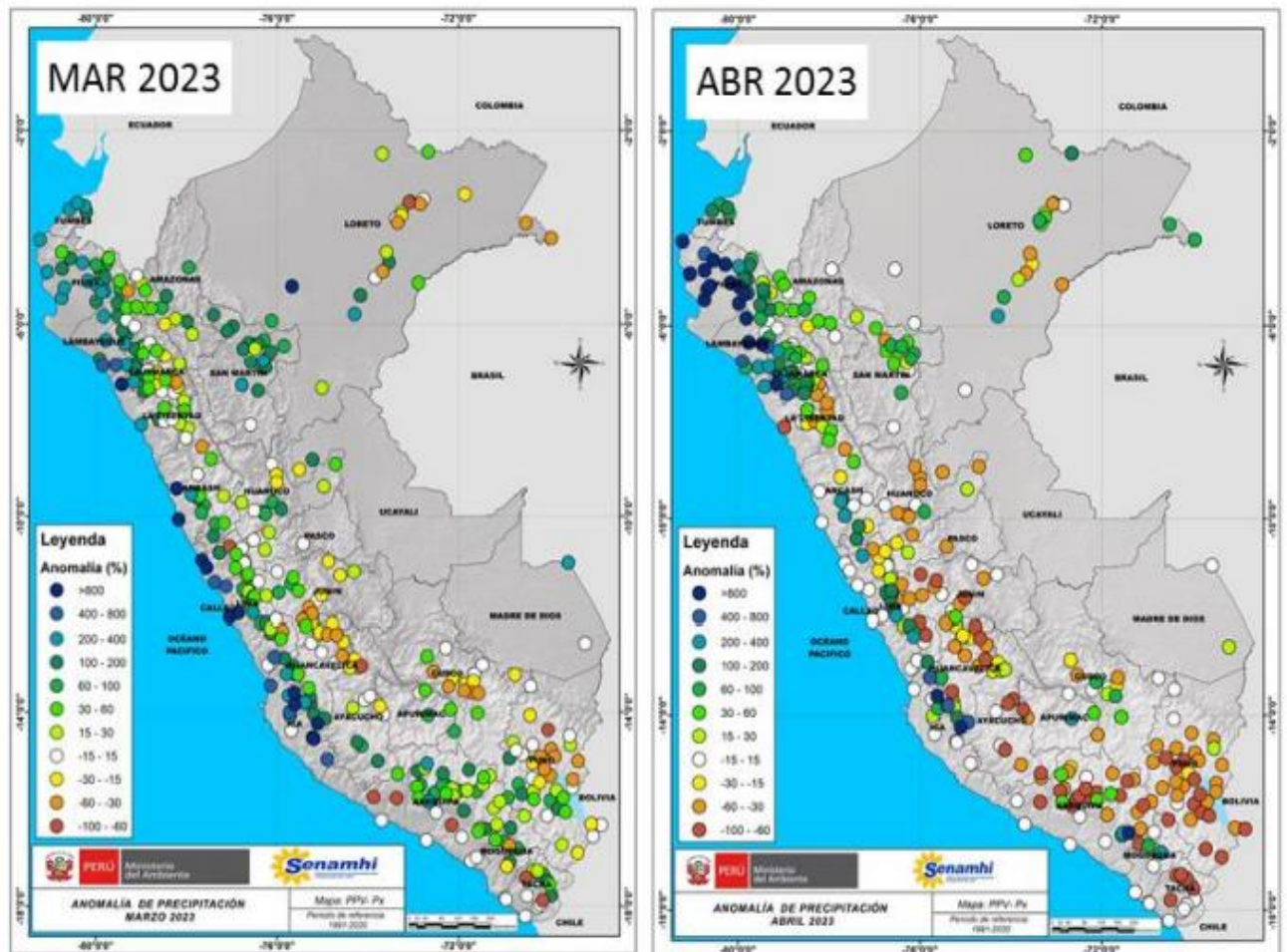
Anomalías de precipitación de marzo -abril, durante El niño costero 2023
