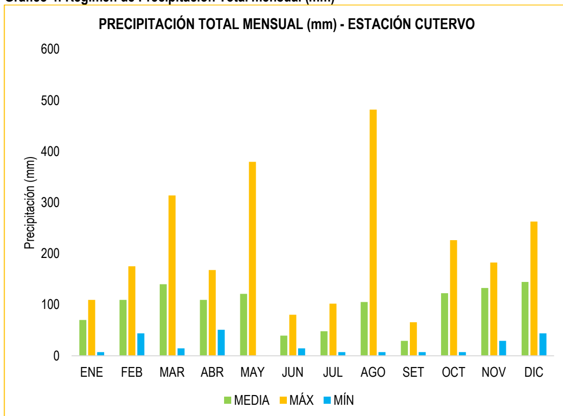
Gráfico 4: Régimen de Precipitación Total mensual (mm)
