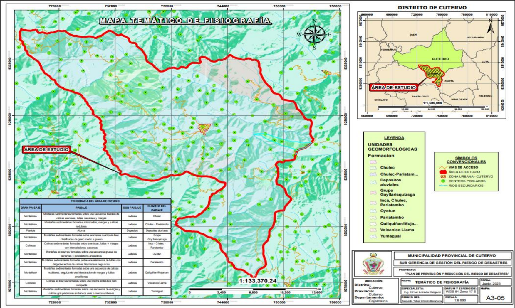
Figura 11: Mapa de Fisiografía del área de estudio
