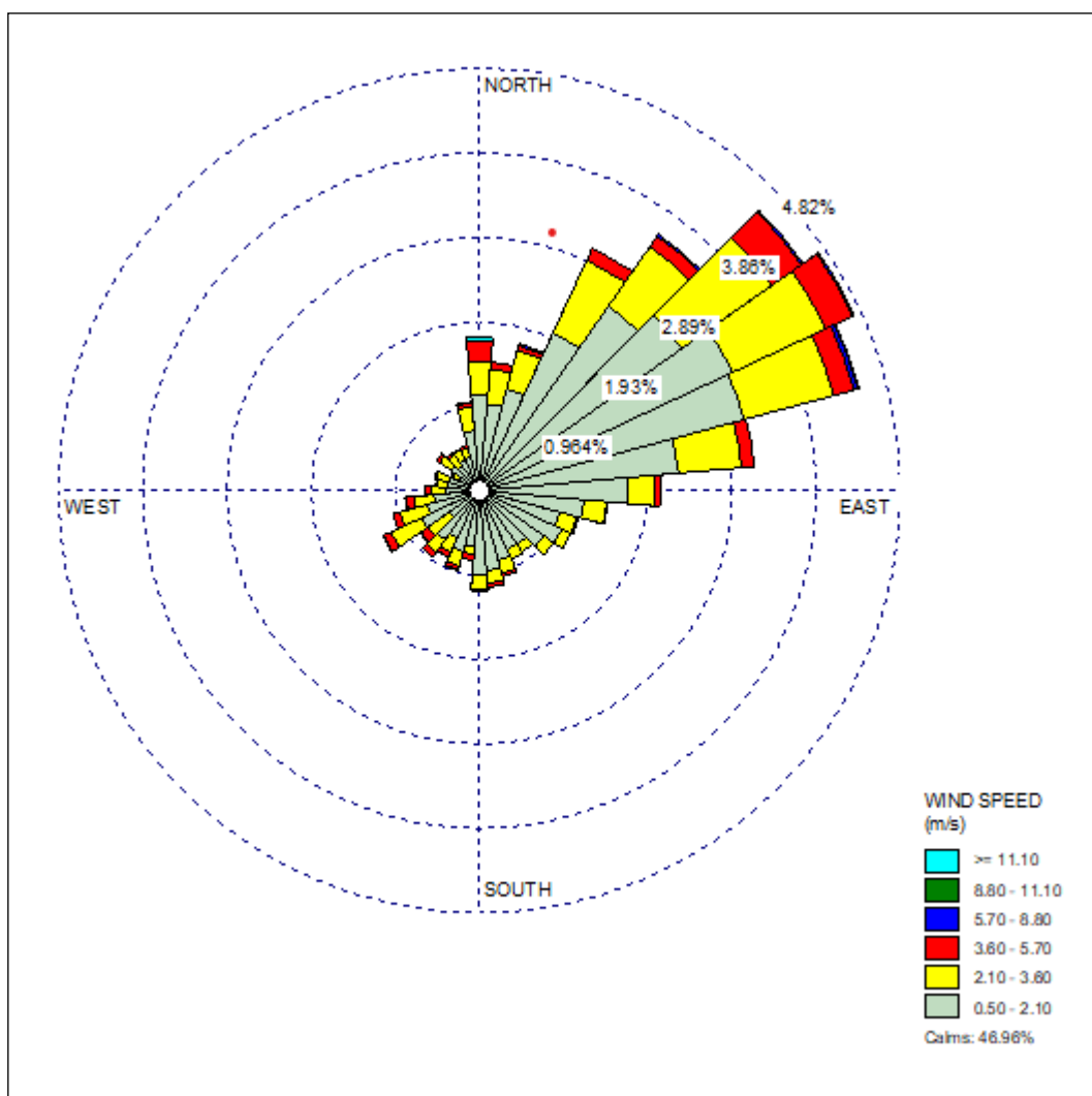
Figura 8: Rosa de viento, estación automática meteorológica – Cutervo
