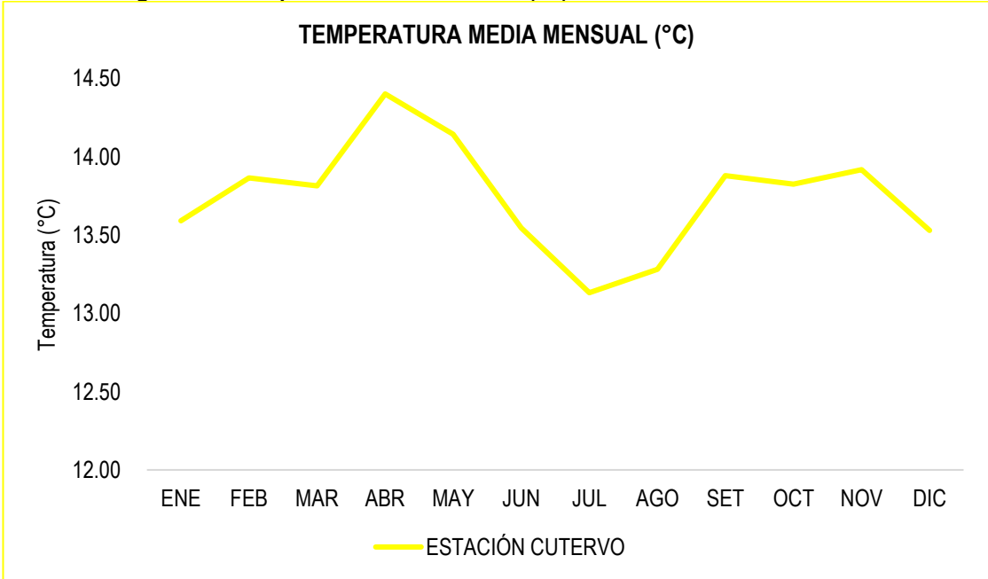
Gráfico 5: Régimen de Temperatura Media Mensual (°C)
