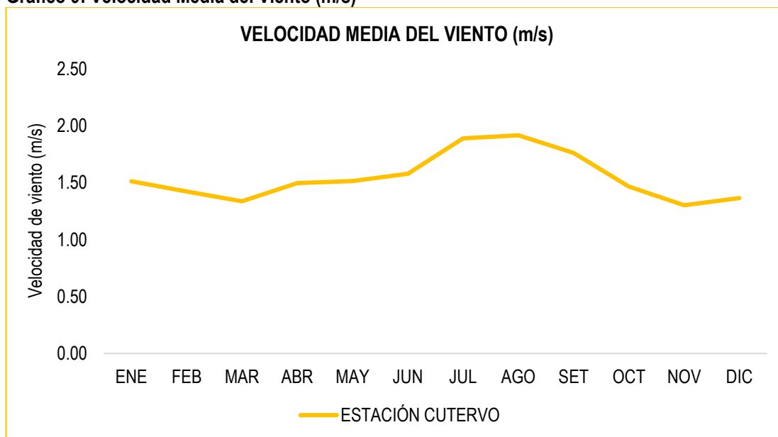
Gráfico 9: Velocidad Media del Viento (m/s)
