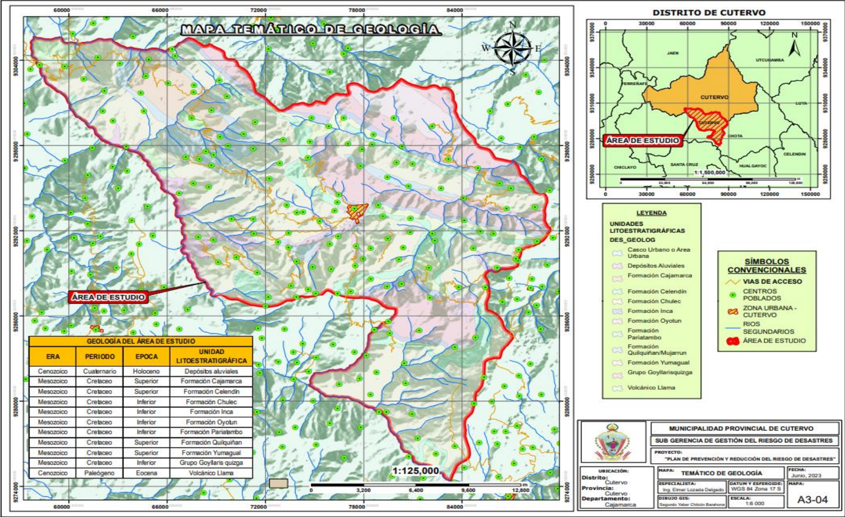
Figura 10: Mapa de Geología del área de estudio.
