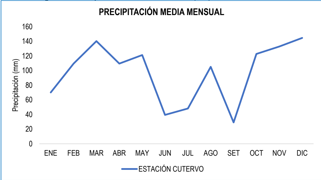
Gráfico 3: Régimen de Precipitación Total Media Mensual (mm)
