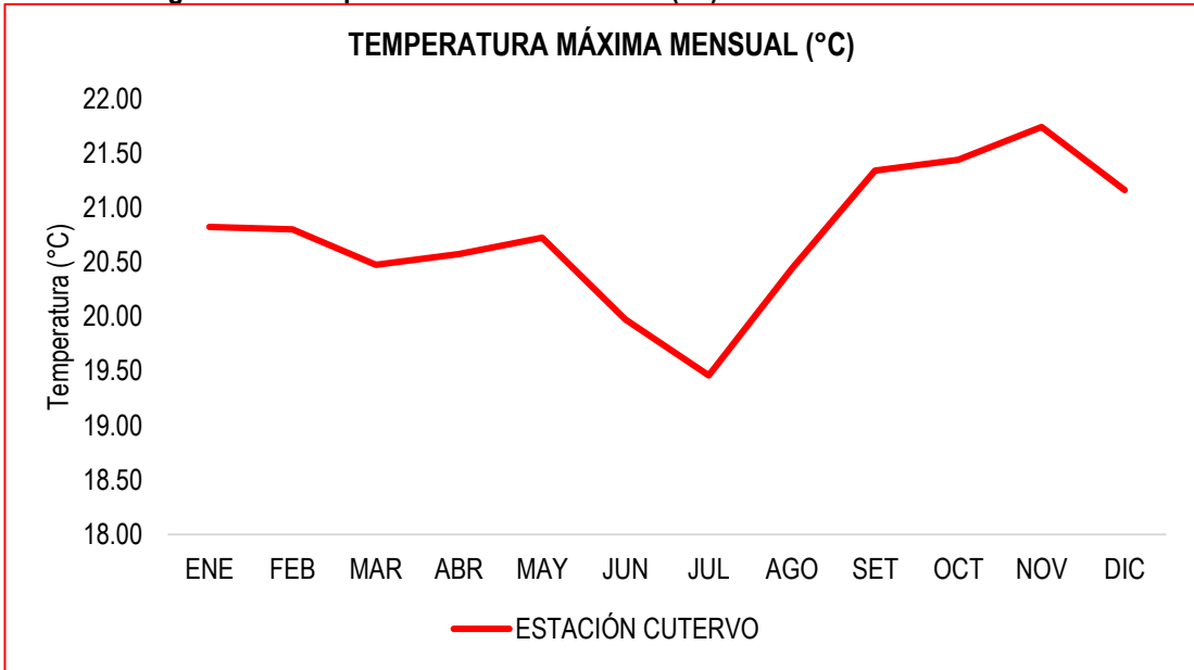
Gráfico 7: Régimen de Temperatura Máxima Mensual (°C)
